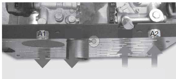
A1 = Polazni vod 3/4 " M A2 = Povratni vod 3/4 " M
