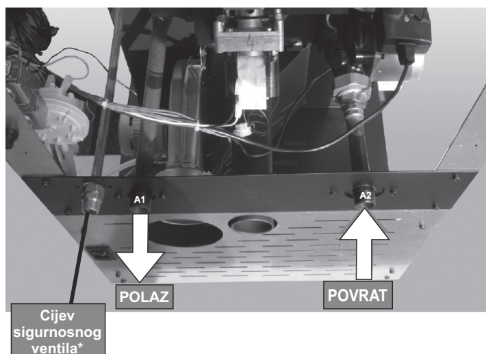
A1 = Polazni vod 3/4 " M A2 = Povratni vod 3/4 " M
