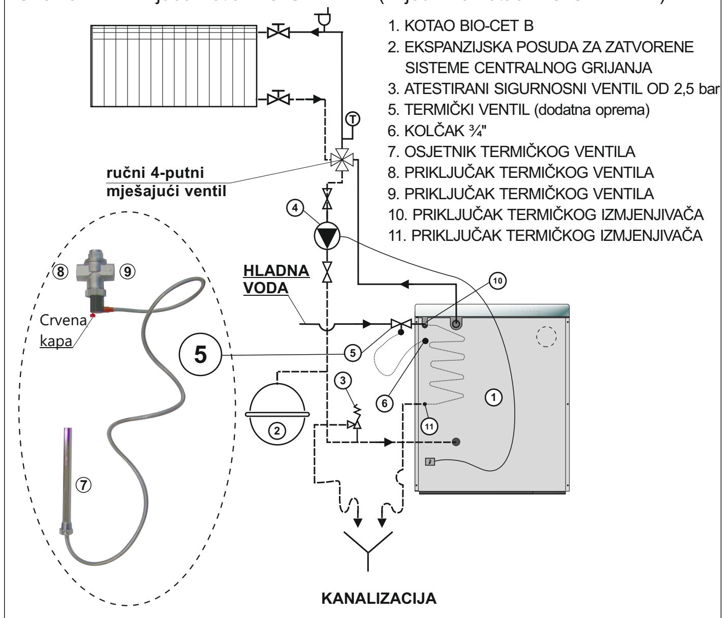
Shema 2. - Priključci kotla BIO-CET B - L (vrijedi i za kotao BIO-CET B - D)
