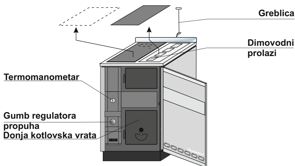
Slika 7. Čišćenje površina - BIO-CET B-L (vrijedi i za kotao BIO-CET B - D)
