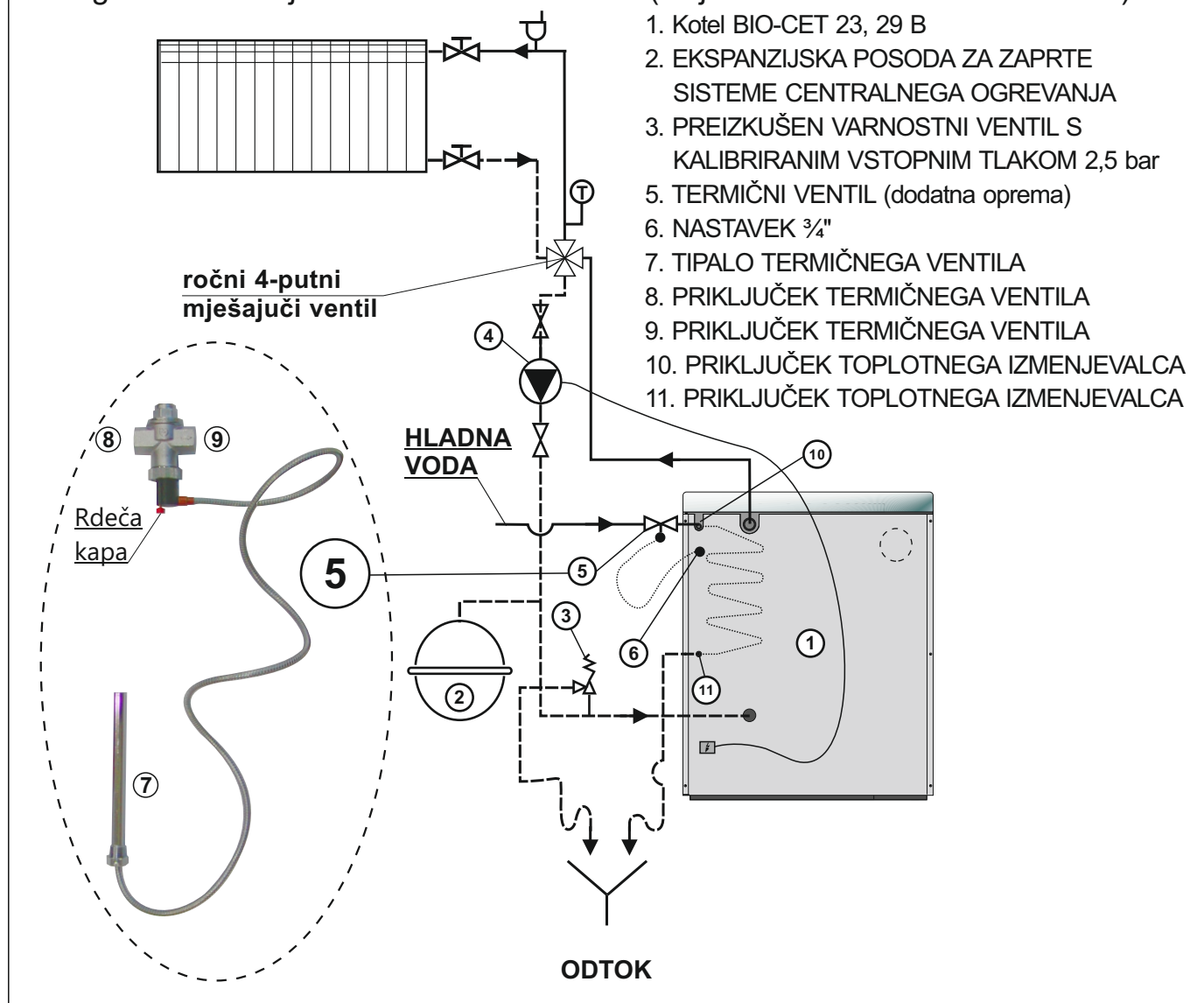
Diagram 2. - Priključki kotla BIO-CET B - L (velja tudi za kotel BIO-CET B - D)
