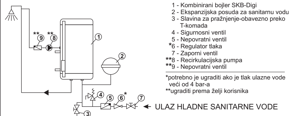
Shema 1. Ugradnja kombiniranog bojlera SKB-Digi na vodovodnu instalaciju
