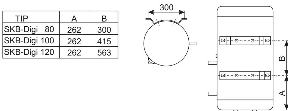
Slika 3. Montaža kombiniranog bojlera SKB-Digi na zid
