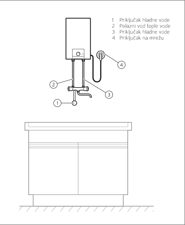
Ugradnja iznad izljevnog mjesta
