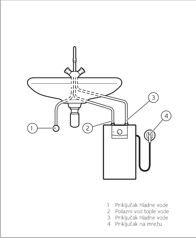
Ugradnja ispod izljevnog mjesta
